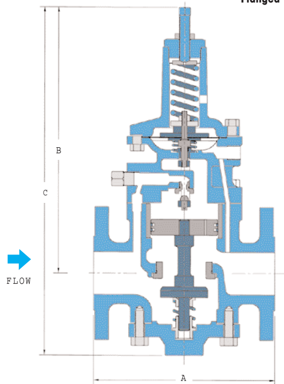
402/403 Flanged
